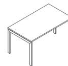
BOU20 1400 / 800 / 740 38.3 kg
